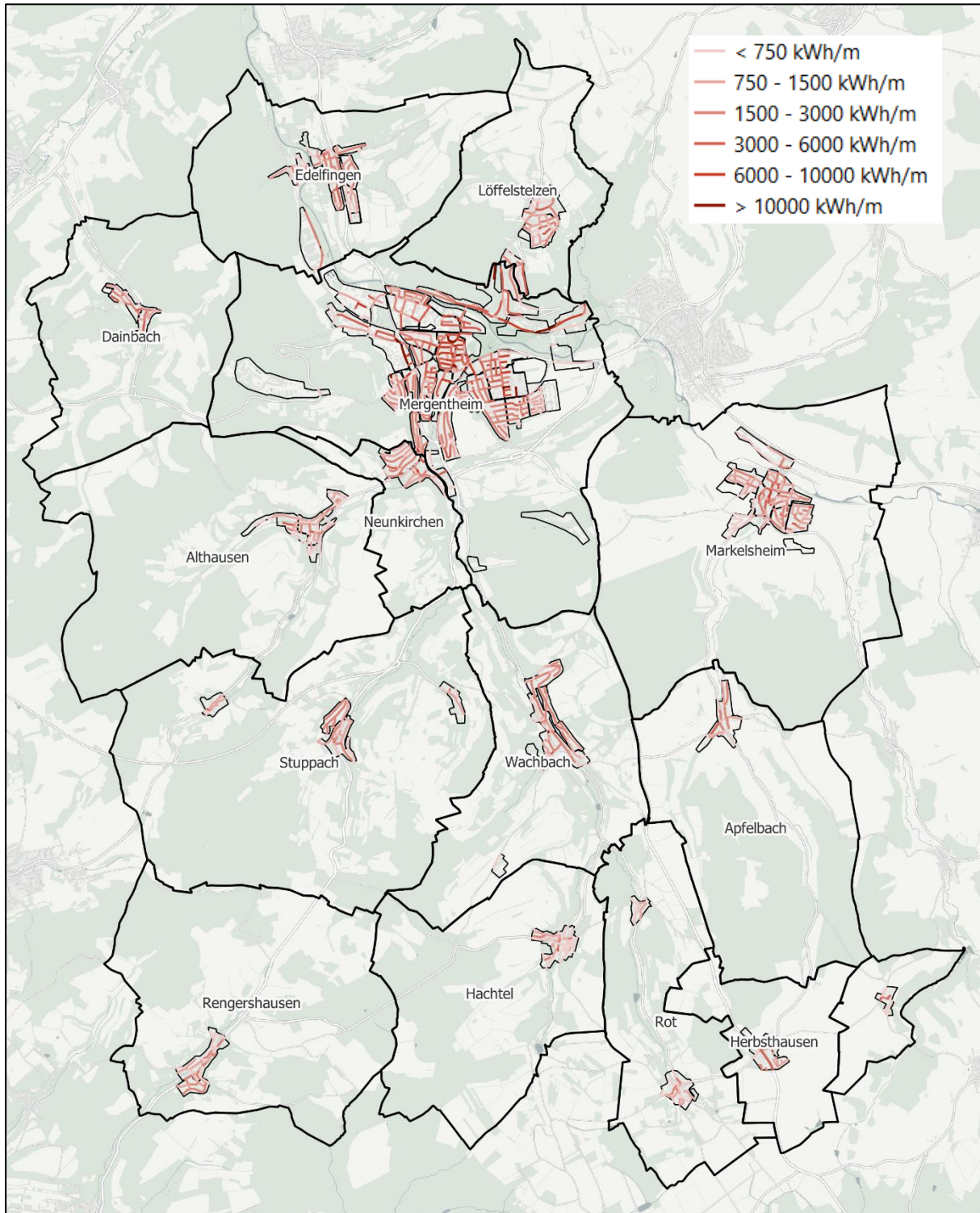
Abbildung 7: Wärmelinienindichte
