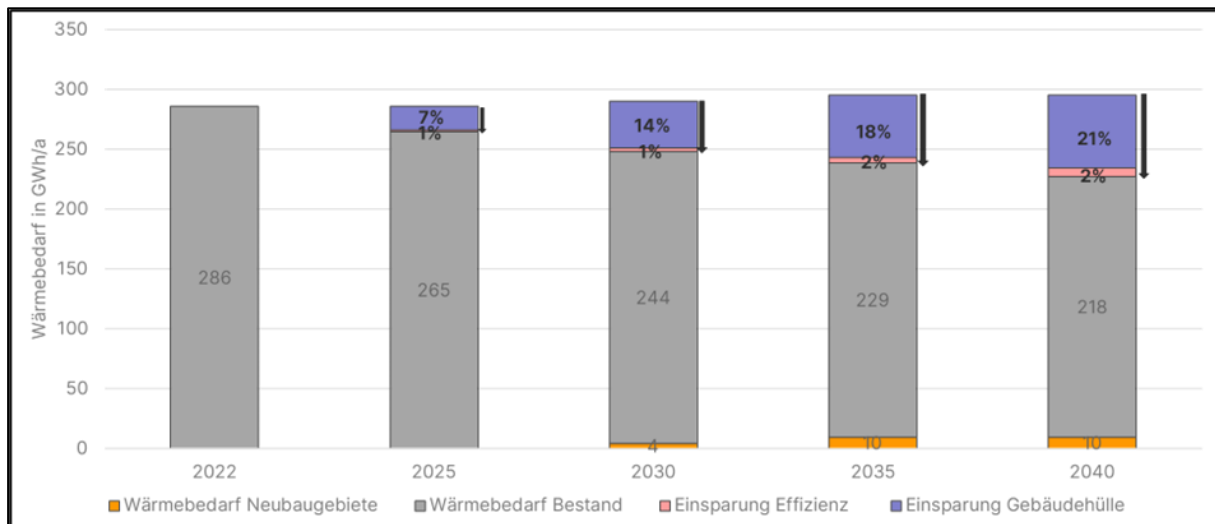
Abbildung 11: Energiebedarfsentwicklung – Szenario 1
