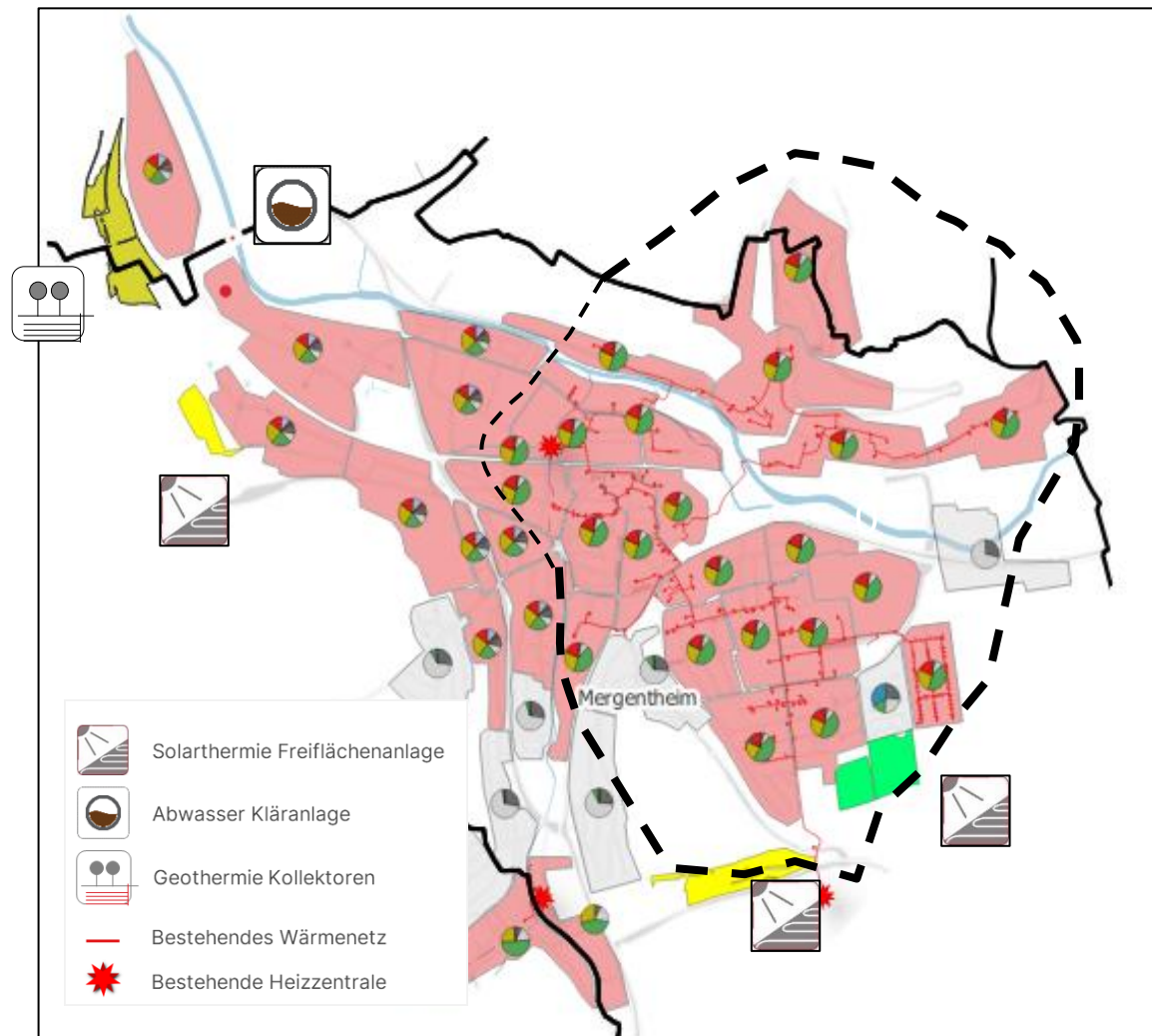
Abbildung 40: Bestandswärmenetz Mergentheim
